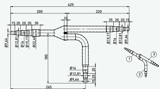
Vloeistofleiding
