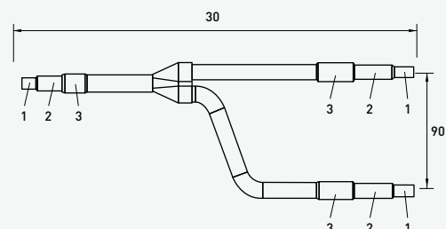
Vloeistofleiding
